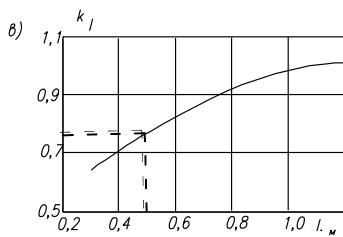
Черт. 1. Значение переходных коэффициентов k а – для положительных изгибающих моментов; б – для отрицательных изгибающих моментов; в – график для определения поправочного коэффициента k к одному коэффициенту k
