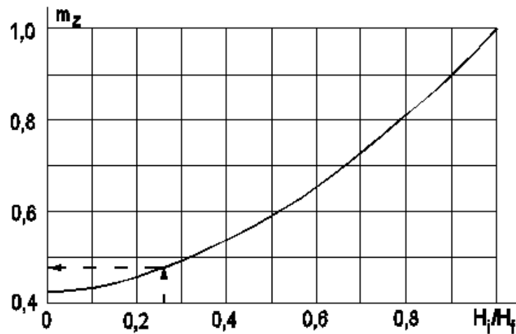
Г.2-сызба. m_z коэффициентін анықтауға арналған кесте
