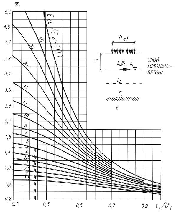
Черт. 9. Номограмма для определения удельных растягивающих напряжений при изгибе \bar{S}_r в асфальтобетоне
