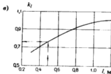
1-сызба. k_i ауыспалы коэффициентінің мәні а – жағымды иілім сәттер үшін; б – теріс иілімді сәттер үшін; в – k_i ауыспалы коэффициентіне k_1 түзету коэффициентін анықтау үшін кесте;
