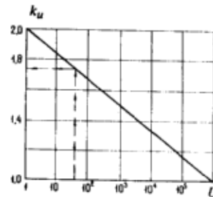
3-сызба. k_u коэффициенттерін анықтау үшін кесте.
