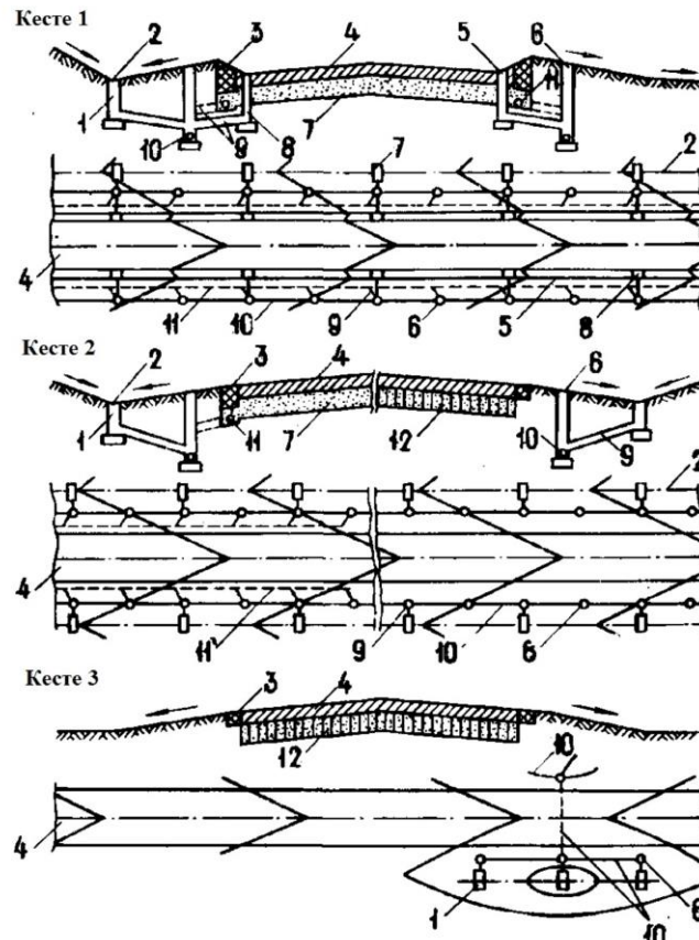
5-сурет - Аэродромның суды қашыртқы және дренаждық кестелері (көлденең профилі және жоспар)
