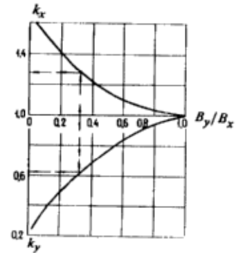
2-сызба. Ортотропты тақталарда ішкі күшті қайта бөлуді есепке алатын k_x және k_y коэффициенттерін анықтау үшін кесте.
