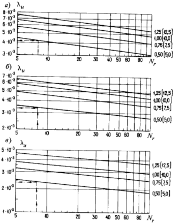
8-сызба. Топырақтарда салынатын қатты емес аэродромдық жабындылардың \lambda_u шектік салыстырмалы иілімдерді анықтау кестесі.
