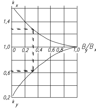
Черт. 2. График для определения поправочных коэффициентов k_x и k_y учитывающих перераспределение внутренних усилий в ортогональных плитах
